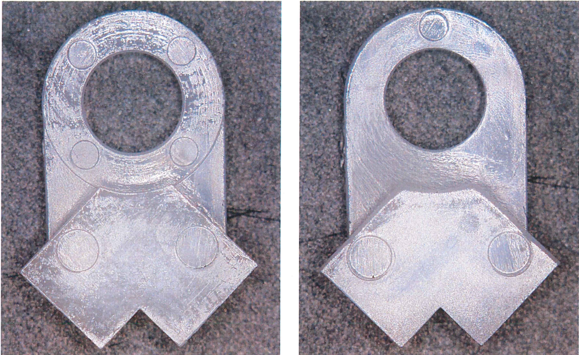
写真1. 突き出しピン位置の比較画像(左:旧製品 右:新製品)
