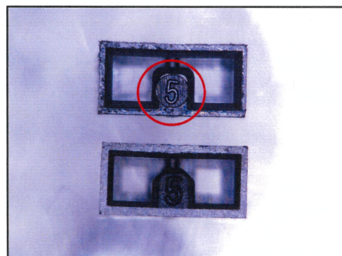
②上面形状 上側 増設金型 下側 従来金型
