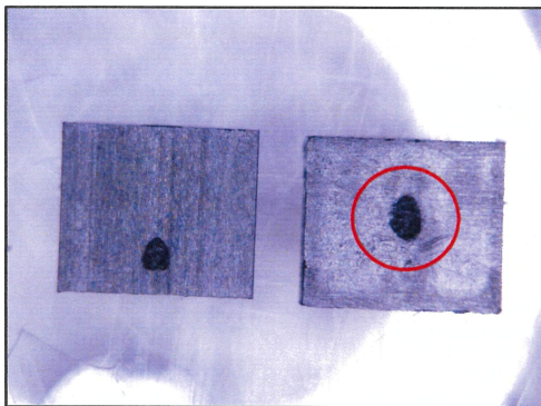
①側面(ゲート側:材料注入位置) 左側 従来金型 右側 増設金型
