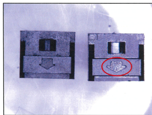
④側面(矢印側) 左側 従来金型 右側 増設金型
